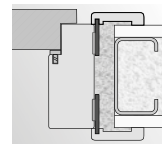
beépítés a pürhabbal kőműves falba
