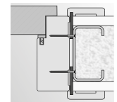
beépítés csavarokkal gipszkarton falba
